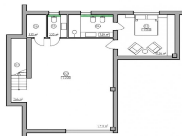
PLANTA SÓTANO 96 m 2
