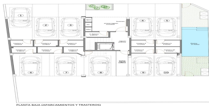
10 VIVIENDAS, TRASTEROS Y PISCINAS
