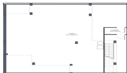
PLANTA SÓTANO
